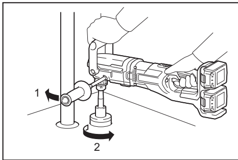
▶ 1. 반동 2. 역방향
