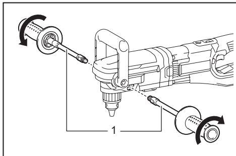
▶ 1. 사이드 그립
