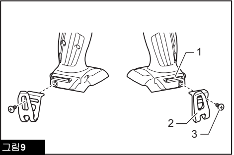
그림9 1. 홈 2. 갈고리 3. 나사
