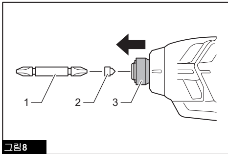
그림8 1. 드라이버 비트 2. 비트 피스 3. 슬리브
